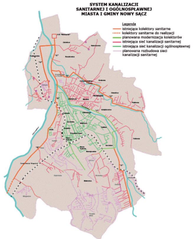
Rys. 1. | Schemat kanalizacji Nowego Sącza
